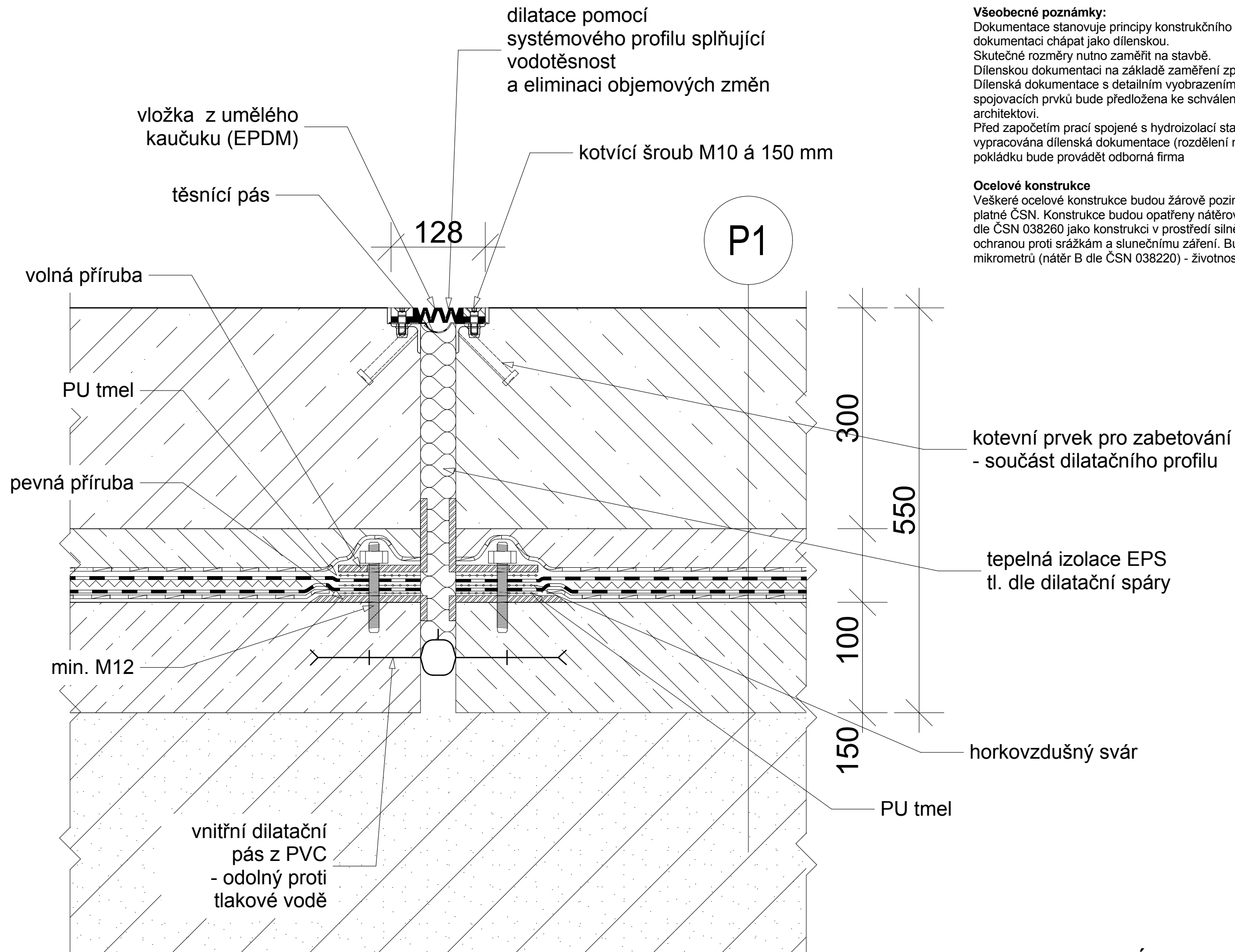
D.14 - DETAIL PODLAHOVÉ DILATACE (betonový kryt) M1:5
