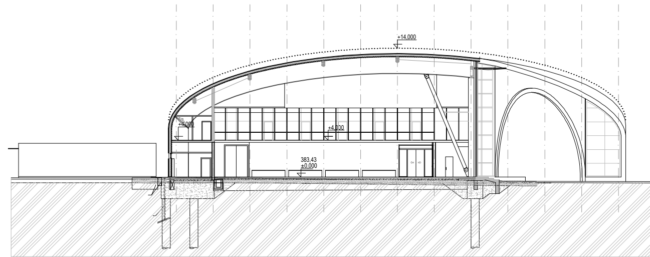
Řez F
