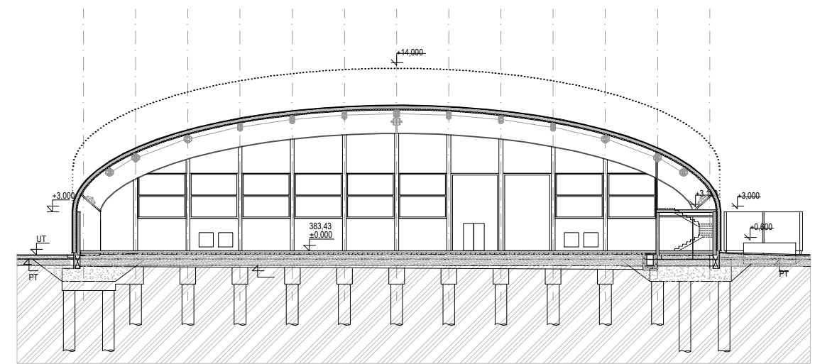
Řez D
