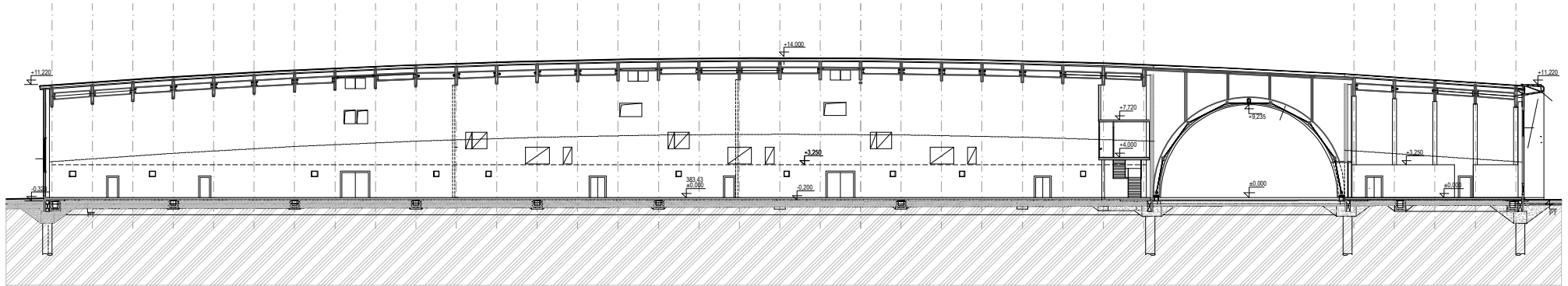
Řez A
