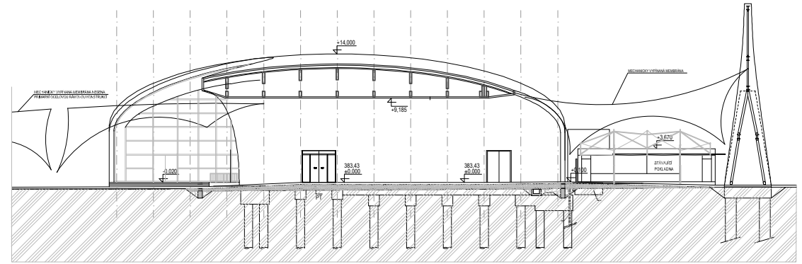
Řez E
