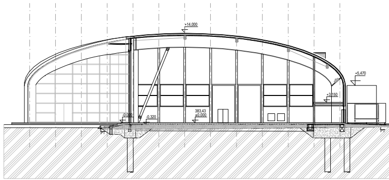
Řez B
