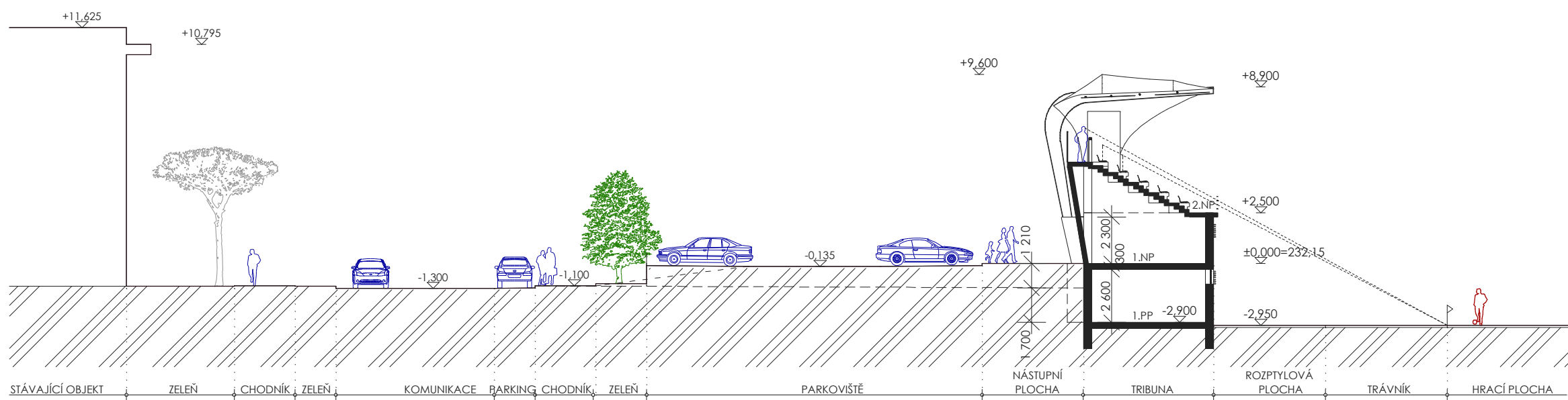
PŘÍČNÝ ŘEZ TRIBUNOU SE ZÁZEMÍM
