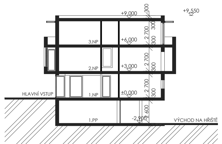
PŘÍČNÝ ŘEZ SPORTOVNÍ UBYTOVNOU
