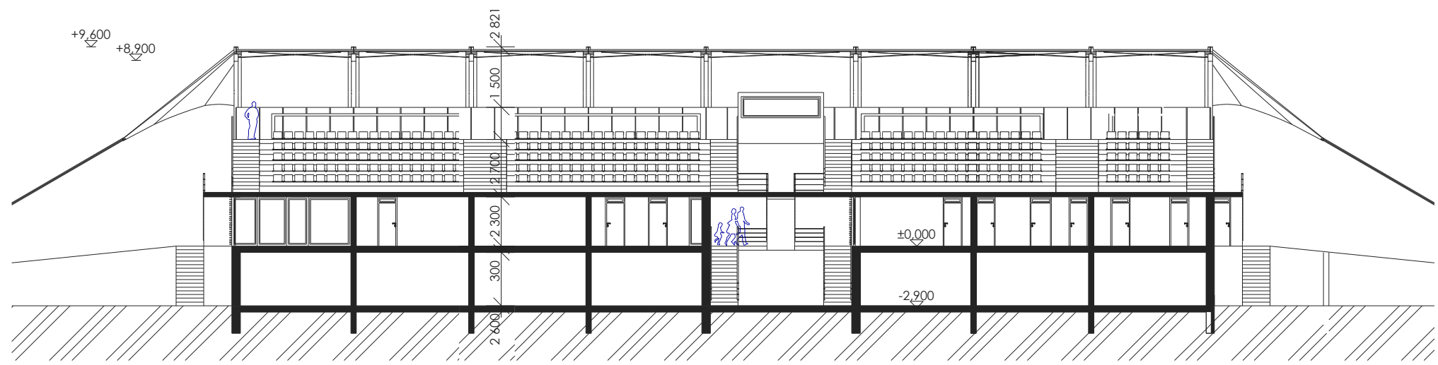
PODÉLNÝ ŘEZ TRIBUNOU SE ZÁZEMÍM
