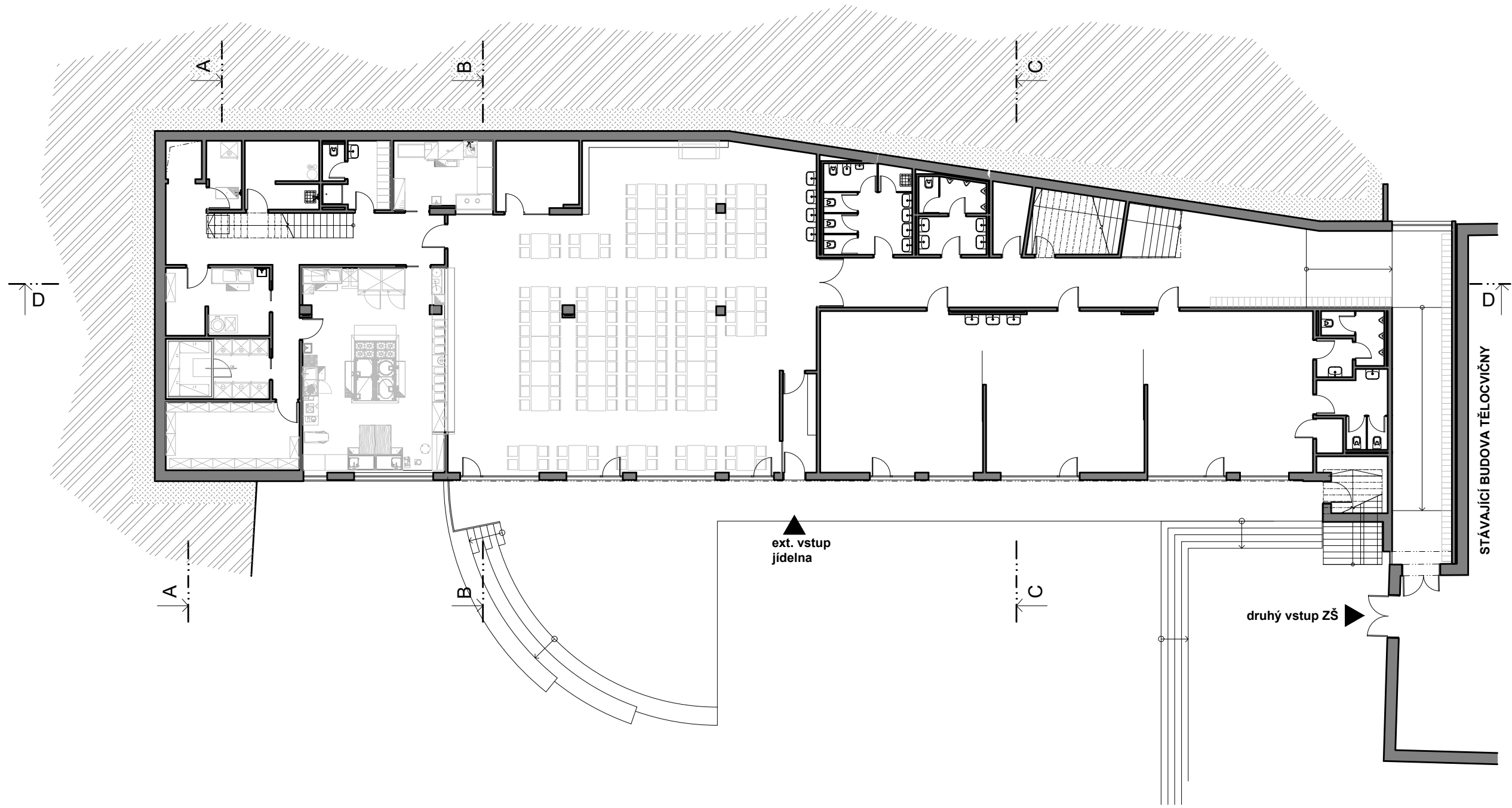
PŮDORYS 1.PP
